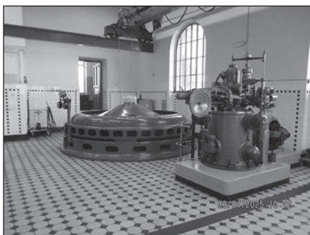
Francisova turbína
