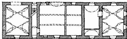
Borovnice - skica půdorysu přizemí špýcharu. 1984.
