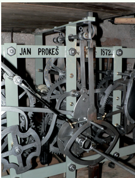
Zrestaurovaný stroj
