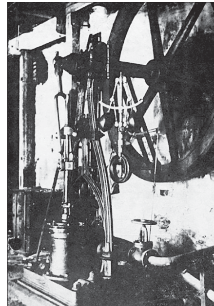
Archivní fotografie parního stroje z Chlumecké strojírny (ze sbírky NTM)
