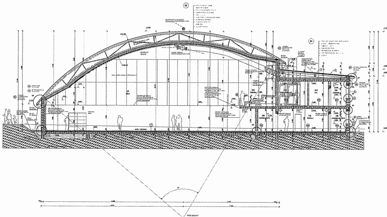
Řez halou z pohledu od malých závor.
