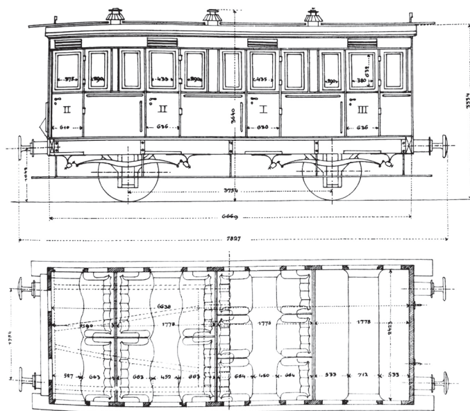
Osobní vůz Pardubicko-liberecké dráhy z roku 1858. Zleva jeden a půl oddíl II. třídy o celkovém počtu 12 míst, uprostřed oddíl I. třídy se šesti křesly a napravo třetí třída s dřevěnými lavicemi. Vozy IV. třídy byly bez lavic.
