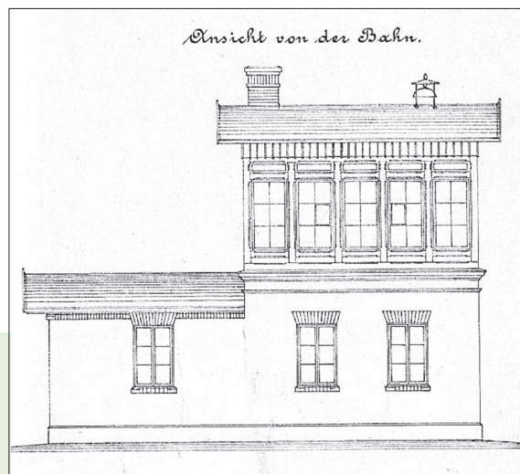
Výkres patrového stavědla č. 2 nacházejícího se na liberecké straně nádraží. Odtud byly výhybkářem přestavovány výhybky na přilehlé části kolejíště.
