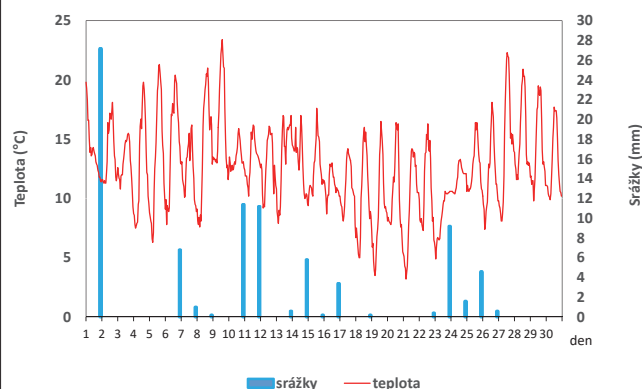
Teploty vzduchu 200 cm nad zemí a srážky v areálu VS Opočno v září 2017
