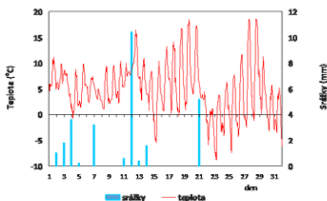
Teploty vzduchu 200 cm nad zemí a srážky v areálu Výzkumné stanice Opočno v březnu 2020
