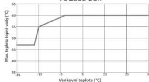
TČ Zuba Dan
