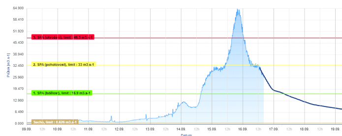
Hronov, tok Metuje, předpovědní profil kategorie B
