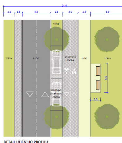
DETAIL ULIČNÍHO PROFILU
