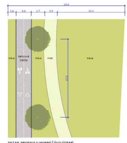
DETAIL PROFILU V HORNÍ ČÁSTI ÚZEMÍ
