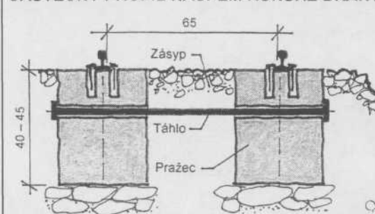
ČÁSTEČNÝ PROFIL NÁSPEM KOŇSKÉ DRÁHY
