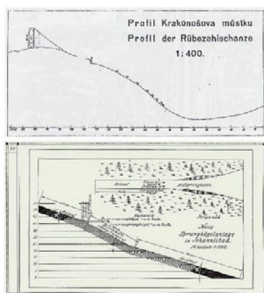
Schematický náčrt profilu Krakonošova můstku a plánec prvního můstku v údolí Černošského potoka / Návštěva při skokanských závodech v roce 1925 (Ve výřezu Adolf Berger a šikmo pod ním jeho chalupa č. p. 16) / Bylo málo sněhu – úprava nájezdu
