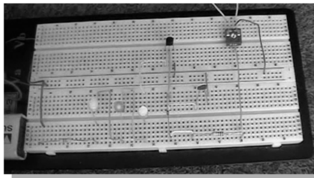
„Barevná hudba“ na nepájivém kontaktním poli
