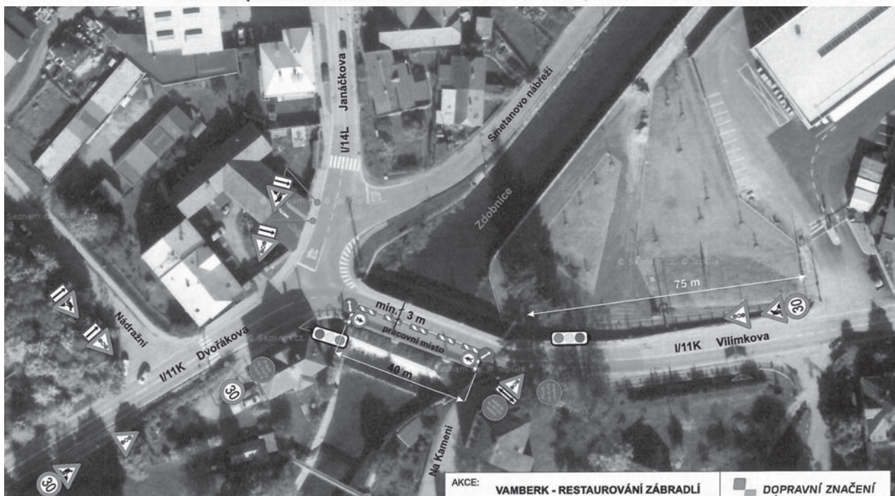
schéma PDZ při restaurování zábradlí mostu - částečná uzavírka pravé poloviny silnice I/11K
