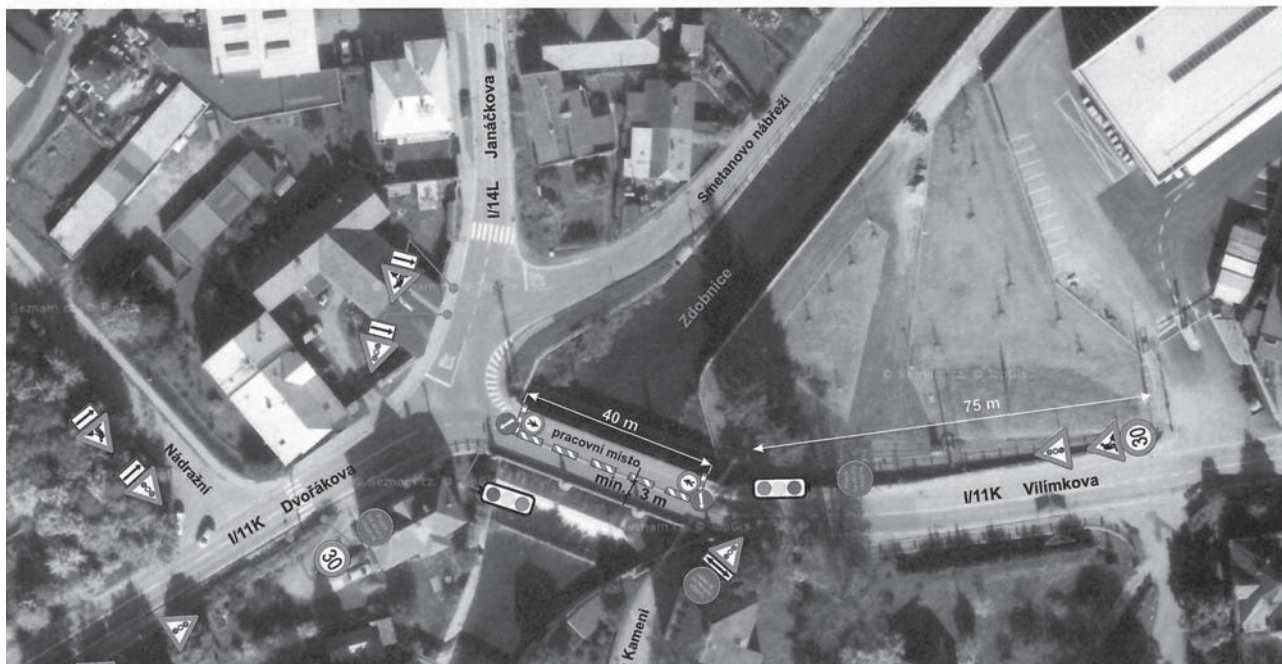
schéma PDZ při restaurování zábradlí mostu - částečná uzavírka pravé poloviny silnice I/11K
