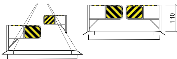
Zábrana vjezdu vozidel - doplnění označení žluté a černé pruhy „Z9“ (oboustranné provedení)
