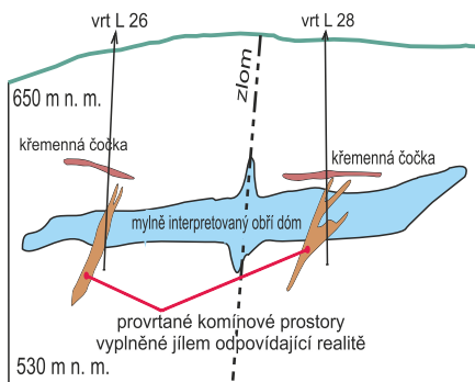
Průřez ložiskem v místě navrtaných dutin.
